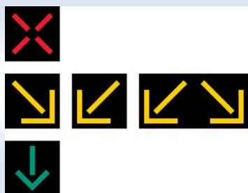
11: Ajokaistaopastin
